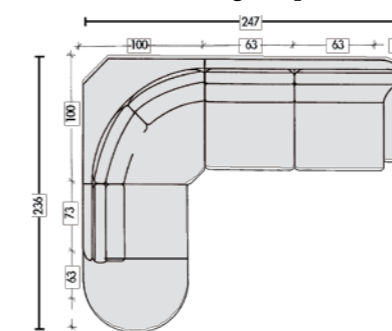
Ecke mit Armlehne 619 Babylon
