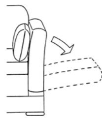
612 Bardelli Klapparmlehne B 18 cm (53 cm abgeklappt) H 72 cm
