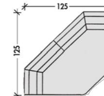
Trapezeckteil B 125 T 125 cm
