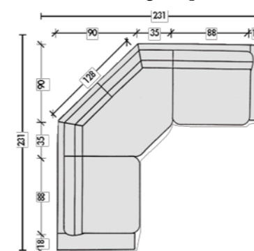
Ecke mit Armlehne 612 Bardelli
